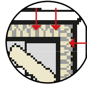
Fuge umlaufend hohlraumfrei mit Dämmstoff ausfüllen
