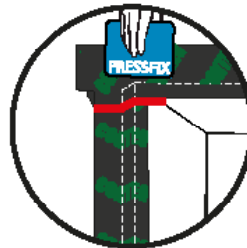
Obere Eckverklebungen herstellen
